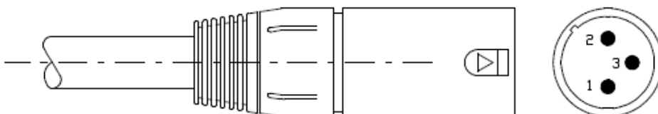
Figur 1 XLR-ladestik
