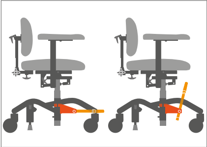
Oppfellbar fotring gir god støtte ved høyere sitteposisjoner. Fotringen felles innunder seteputens framkant.
