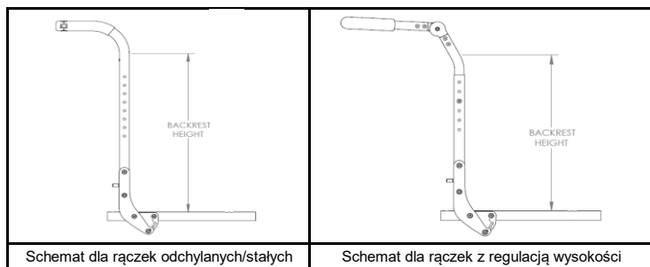
Schemat dla rączek odchylanych/stałych
