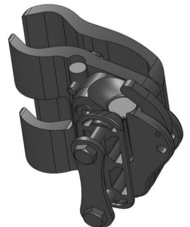
Fixation JAY J3 renforcée (HD) pour une plus grande stabilité
