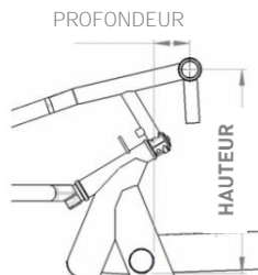
Boîtier de manivelle réglable
