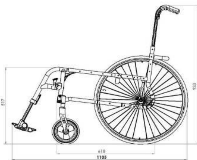
Châssis Swing Away
