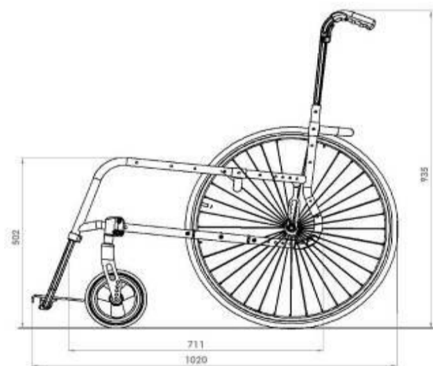
Châssis fixe
