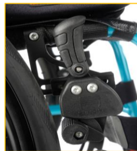
LFE060002 Kniehebelbremse
