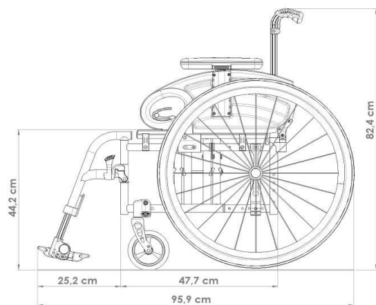
Abbildung: Masse bei Sitztiefe 400 mm und 24" Antriebsräder
