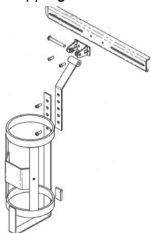
Holder oksygenflaske
