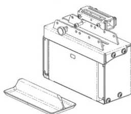
Sikkerhetsboks for armlenemontering
