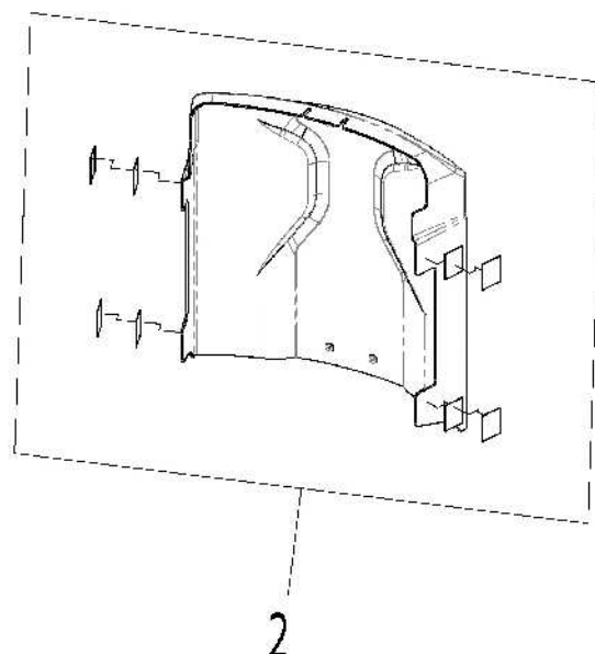
FIXED BACKREST / fester Rücken
