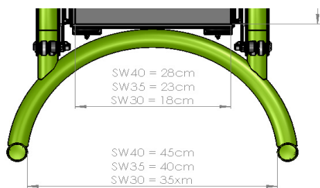
Stol dimensjoner
