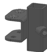
Feste for spesial armlener til 15x15 mm firkantrør
