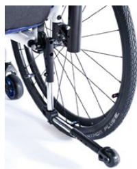
KRF090004 Anti-tip tubes SA
