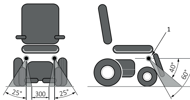
Bevestigingspunten voorzijde
