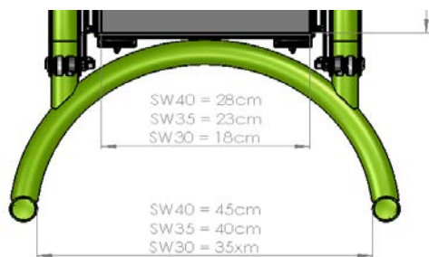
Dimensioni carrozzina
