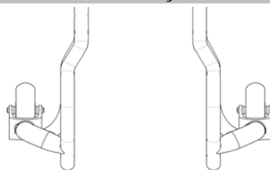
YNG010102 Armação com ângulo p/ exterior (abductor)
