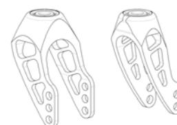
Forqueta de 45 e 32 mm de largura
