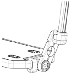
YNG050108 Mecanismo para abatir la plataforma
