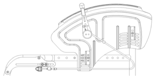
YNG060105 Freno Safari
