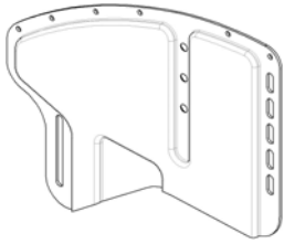
YNG040201 Protector aluminio sin fender
