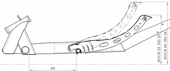
Standardrückenlehne
