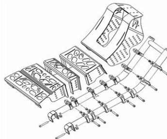
Performance Rückenlehne
