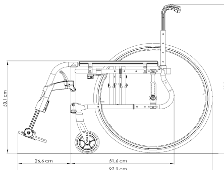
Abbildung: Stuhl mit ST 400 und 24" Rad
