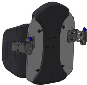
Pontos de ancoragem com desmontagem rápida quick-release
