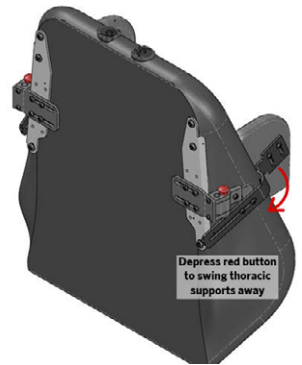
Suportes de tronco reguláveis e abatíveis
