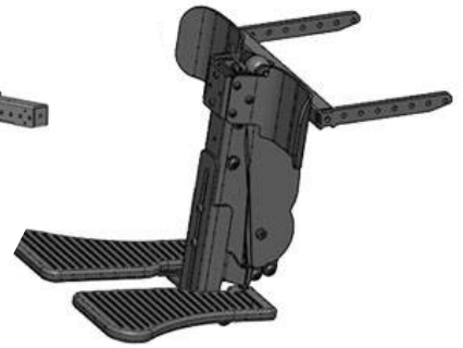
Apoio de pés central elétrico
