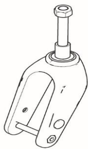
Länkhjulsgaffel 130 mm
